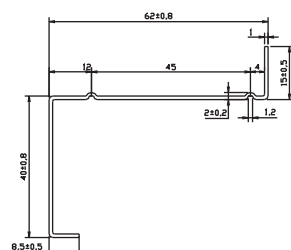
ramka nietłoczona / frame
