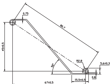
ramka tłoczona / pressed frame
